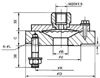
图三( P < 4\text{MPa} )[代号 MF]
