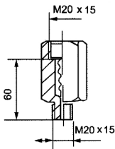
阻尼器 [ZN] 1Cr18Ni9
