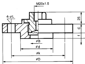
图二( 6\text{MPa} < P < 25\text{MPa} )[代号 MF1]
