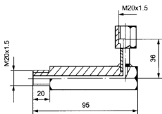
角形接管 [GL]
