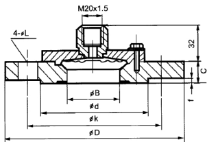
图一( p < 4\text{MPa} )[代号 MF1]
