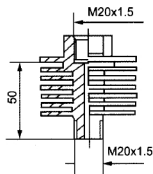
散热器 [SR] 铜镀镍
